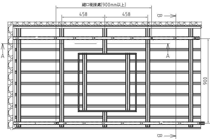
平面組裝示意圖
