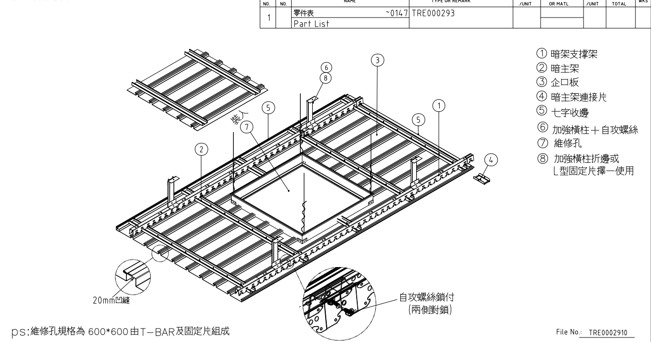
立體組裝示意圖
