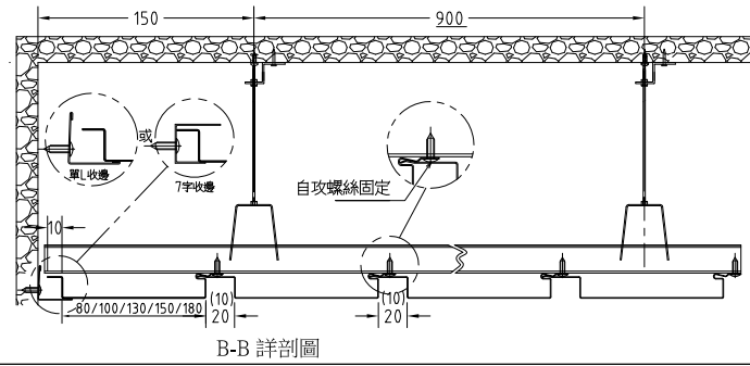
B-B 詳剖圖
