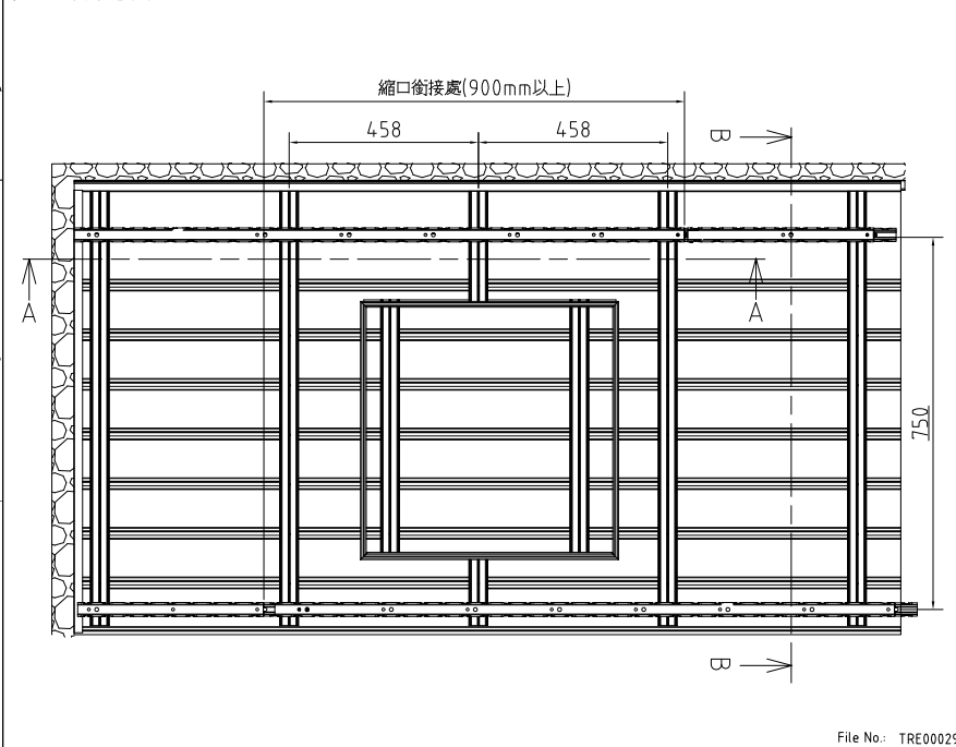
平面組裝示意圖
