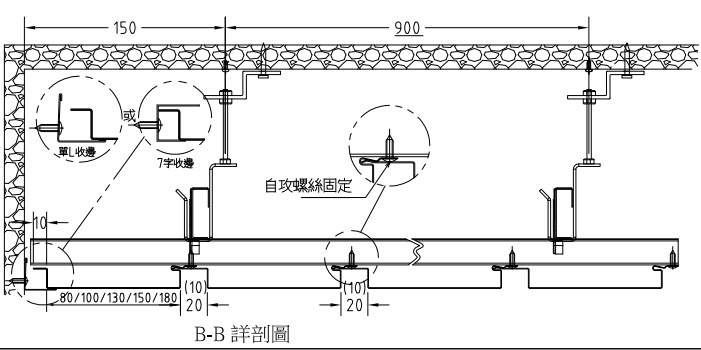
B-B 詳剖圖
