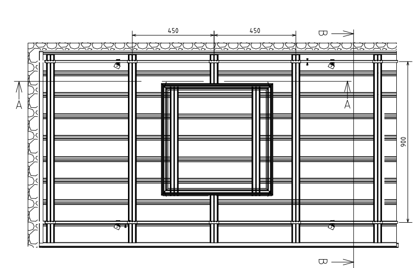
平面組裝示意圖
