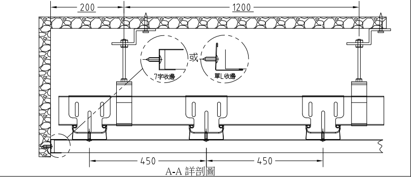
A-A 詳剖圖
