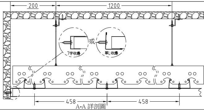
A-A 詳剖圖
